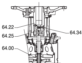
Fig. 6b Pompas gelift, in positie voor borging de pomp as in de koppeling.
