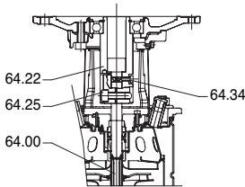
Abb. 6a Stehender Läufer, Welle nicht blockiert in Kupplung
