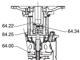
Σχ.6α Σταθεροποίηση ρότορα με ασφαλισμένο άξονα στην σύζευξη. Σχ.6β Ανύψωση ρότορα για ασφαλισμένο άξονα στην σύζευξη.
