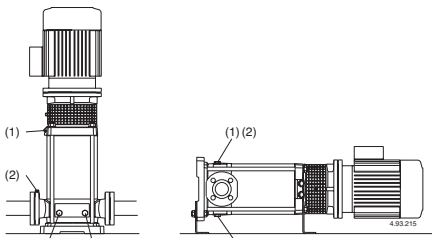
ΕΣΧ. 4 (1) Γέμισμα και εξαέρωση (2) πρόσληψη εξαερισμού (3) Αποστράγγιση
