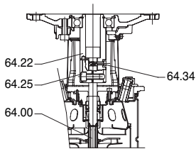
Fig. 6a Rotor apoyado, eje no bloqueado con el manguito,
