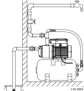
Fig. 2 Funzionamento in aspirazione Suction lift operation Saugbetrieb Fonctionnement en aspiration Funcionamiento en aspiración Sugande funktion Zugsituatie Θέση λειτουργίας με κάθετη αναρρόφηση Работа выше уровня жидкости 负吸水头工作
